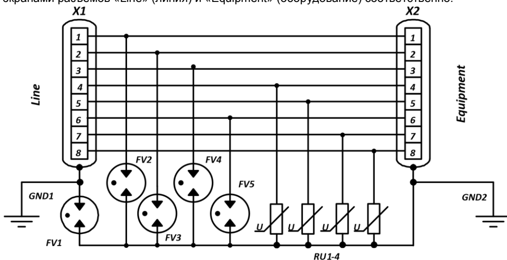
Рис.2 Схема принципиальная.
