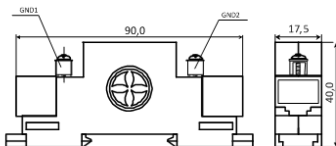
Рис.3 Габариты устройства.
