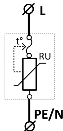
Рисунок 2. Функциональная схема подключения к электроустановке
