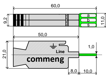
Рисунок 2. Габаритные размеры
