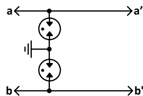
Рисунок 3. Схема электрическая
