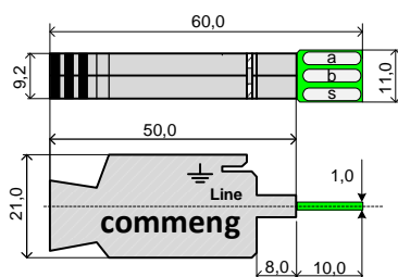
Рисунок 2. Габаритные размеры
