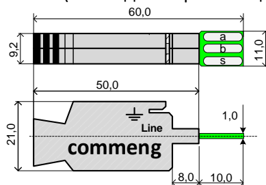
Рисунок 2. Габаритные размеры
