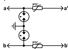
Рисунок 3. Схема электрическая
