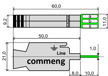
Рисунок 2. Габаритные размеры
