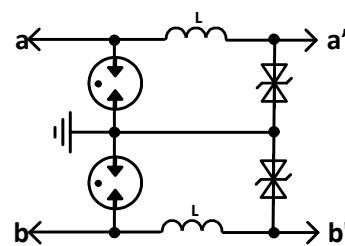
Рисунок 3. Схема электрическая
