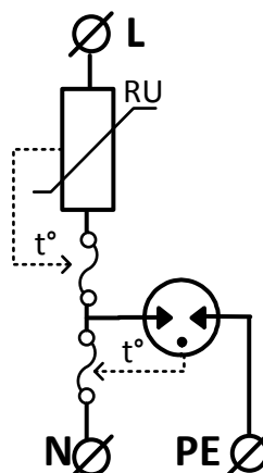
Рисунок 2. Функциональная схема подключения к электроустановке
