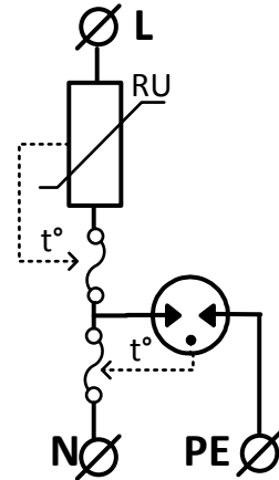
Рисунок 2. Функциональная схема подключения к электроустановке
