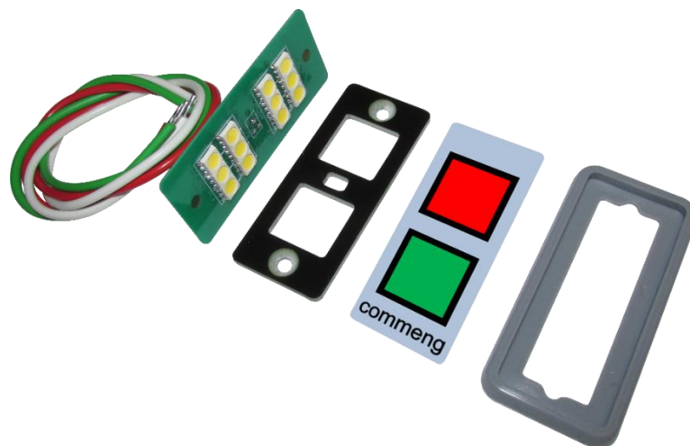
Детали сигнальной панели: плата подсветки, монтажная рамка, защитная пленка, силиконовая прокладка
