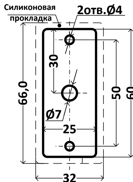
Рисунок 4. Монтажная рамка
