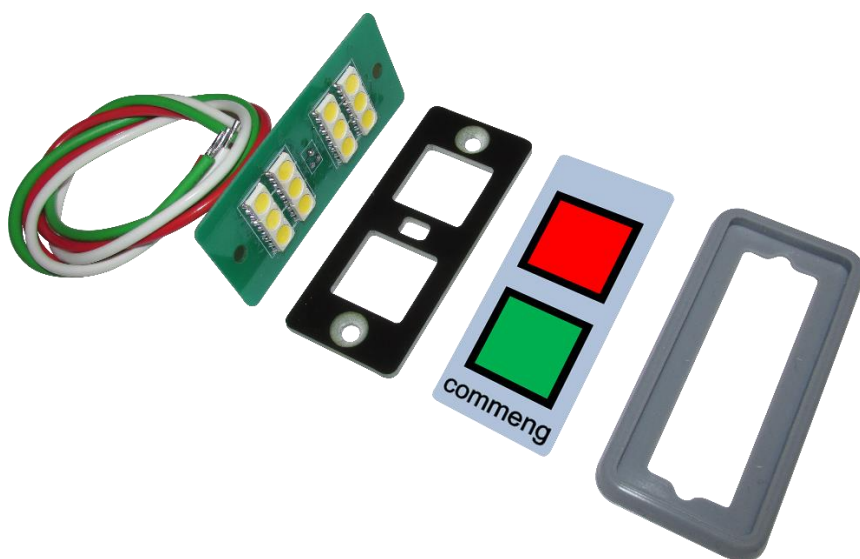
Рисунок 2. Части индикаторной панели: плата подсветки, монтажная рамка, защитная пленка, силиконовая прокладка.
