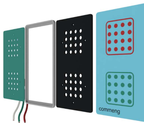
Части индикаторной панели: плата подсветки, монтажная рамка, защитная пленка, силиконовая прокладка
