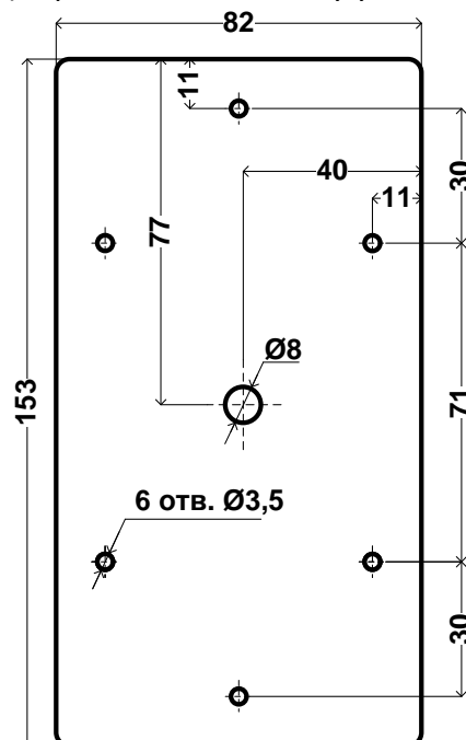
Рисунок 3. Монтажная рамка
