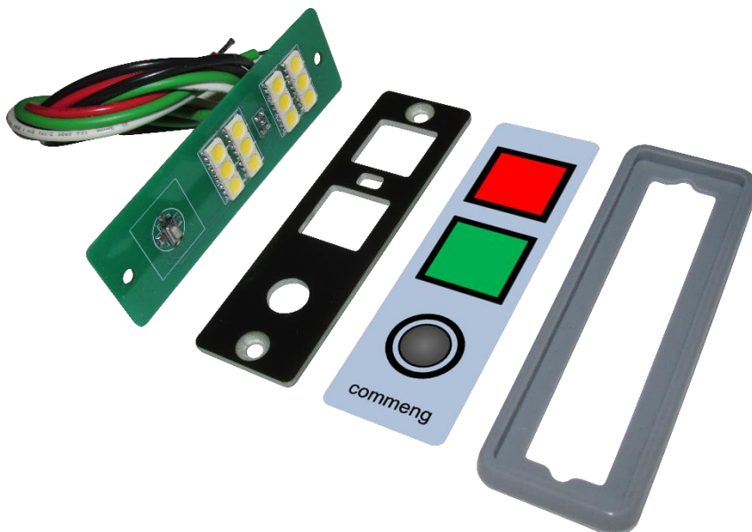
Рисунок 2. Части индикаторной панели: плата подсветки, монтажная рамка, защитная пленка, силиконовая прокладка.
