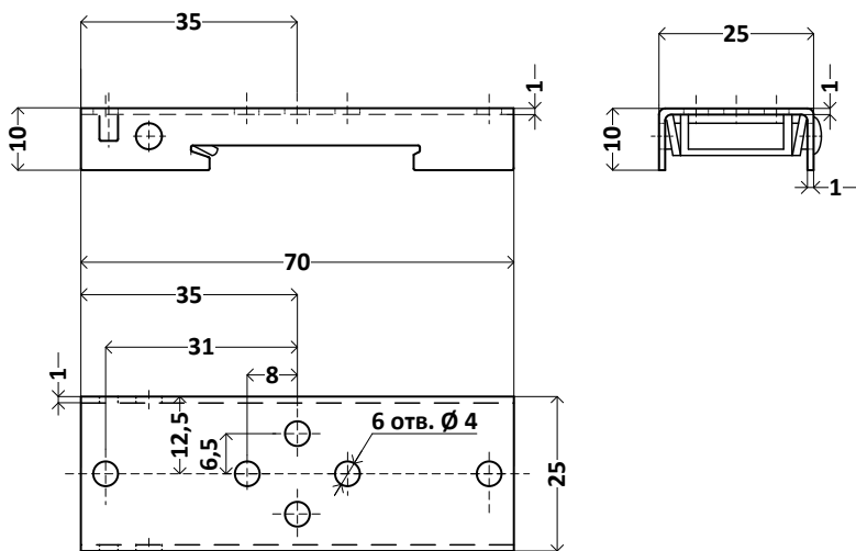
Рисунок 2. Габариты монтажной панели Commeng DR MP
