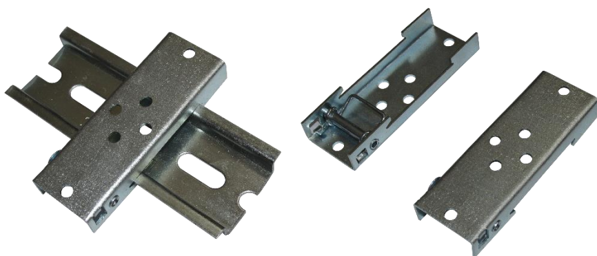
Рисунок 1. Монтажная панель Commeng DR MP
