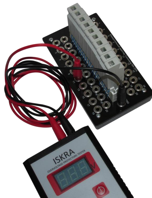
Рисунок 2. Подключение измерительного прибора к устройствам, установленным в плинт
