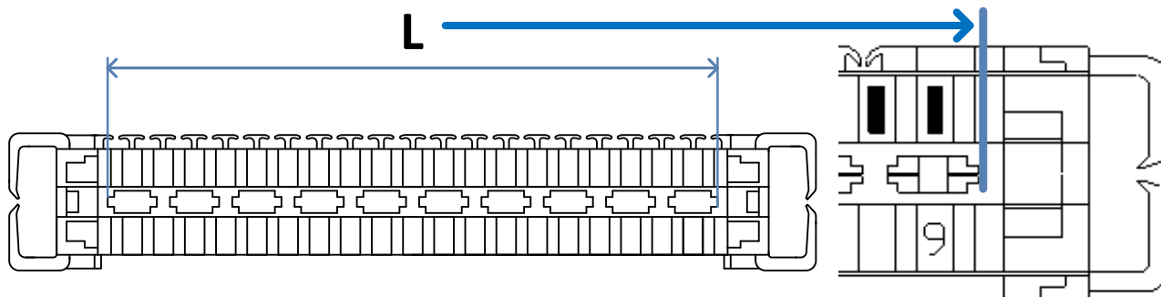
Рисунок 3. Размер 10-парного планты адаптера.
