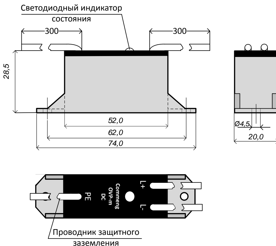
Рисунок 4. Габаритные и установочные размеры устройства OVP-m DC
