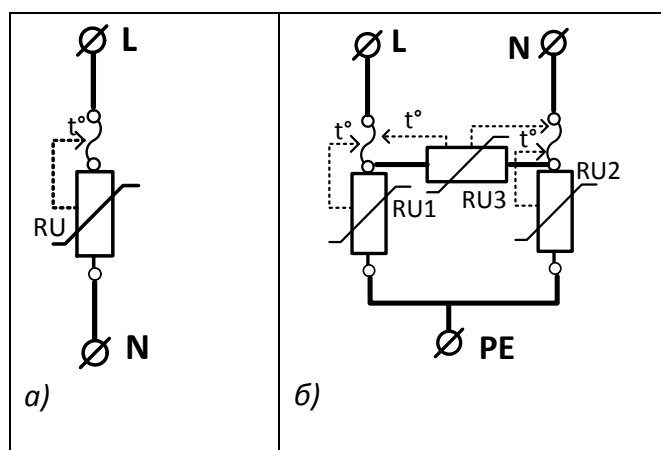
Рисунок 2. Схемы электрические Commeng OVP-m AC 280 (типы устройств см. в табл.2)
