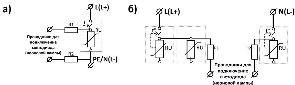
Рисунок 4. Электрические схемы индикации Commeng OVP-m
