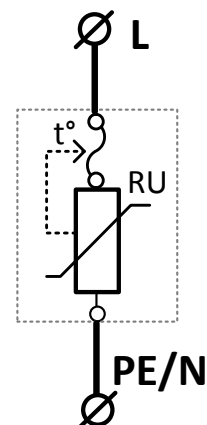
Рисунок 2. Функциональная схема подключения к электроустановке
