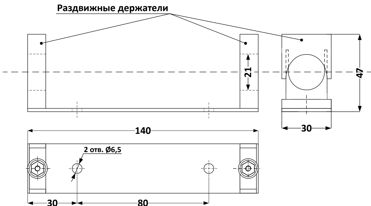
Рисунок 2. Габаритные размеры и установочные размеры основания монтажного ОМ КНУ-2 .
