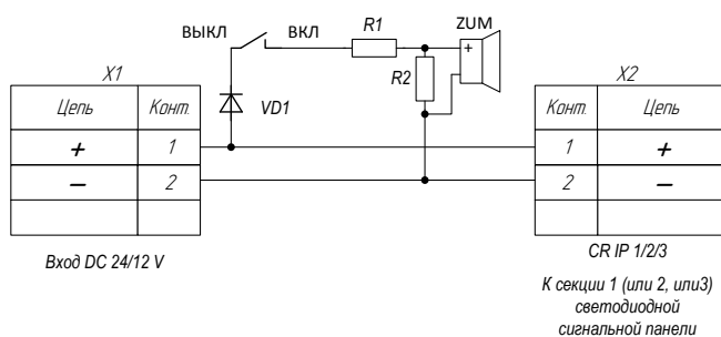
Рисунок 2. Электрическая схема платы звукового сигнала ПЗС-24/12
